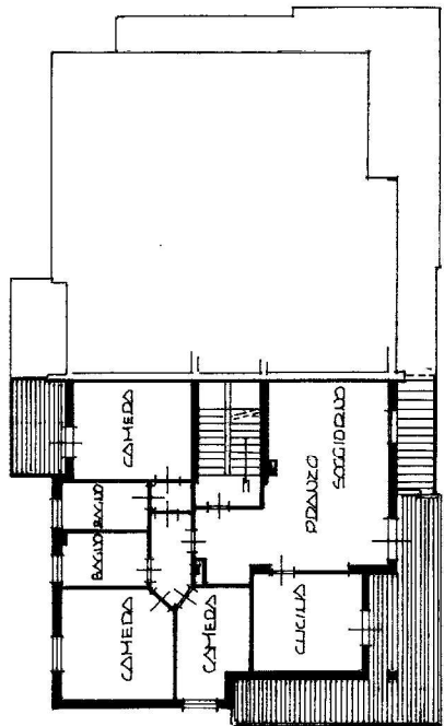
PIANO PRIMO H = mt. 2,90
